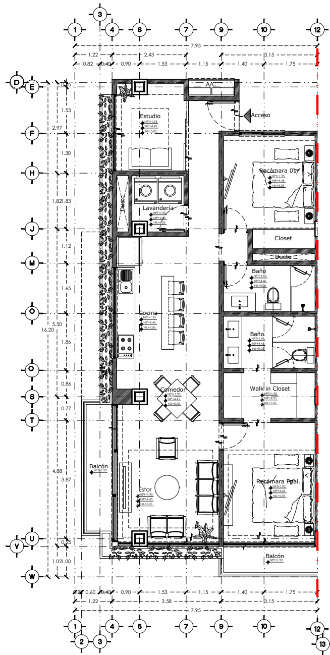
Planta Unidad 01 - Nivel 01 Escala 1 : 1 2 5
